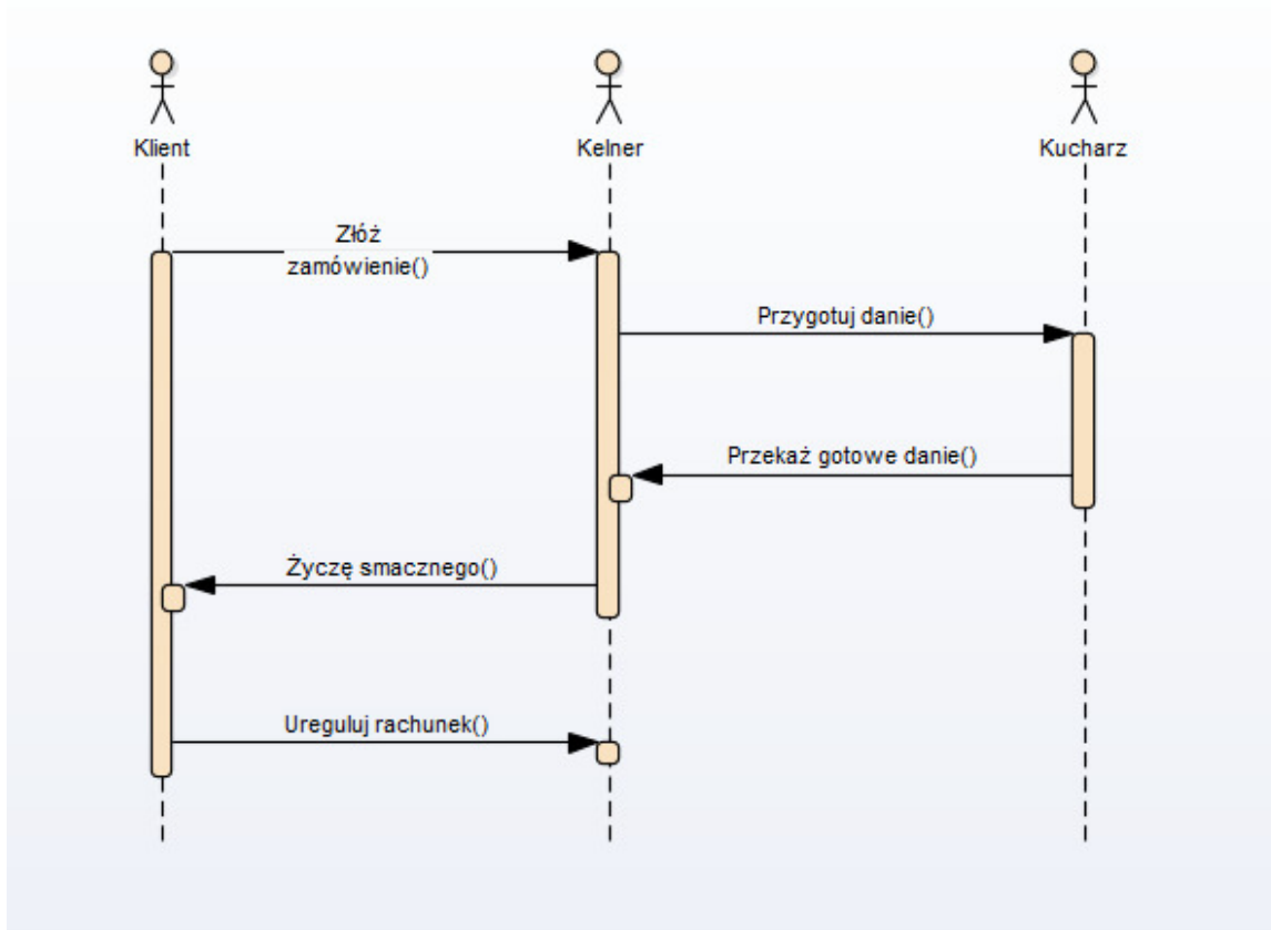
Rysunek 17 - "Restauracja" - przykładowy diagram interakcji
